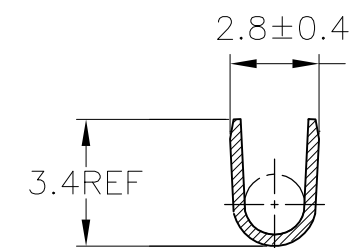
断面 A-A SECT A-A (175030のみ適用) (ONLY 175030)
