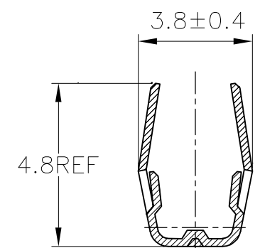
断面 B-B SECT B-B (175030のみ適用) (ONLY 175030)
